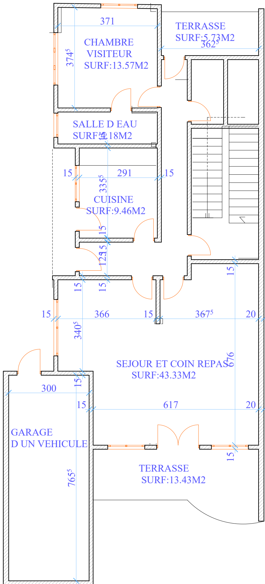
VUE EN PLAN DU RDC
